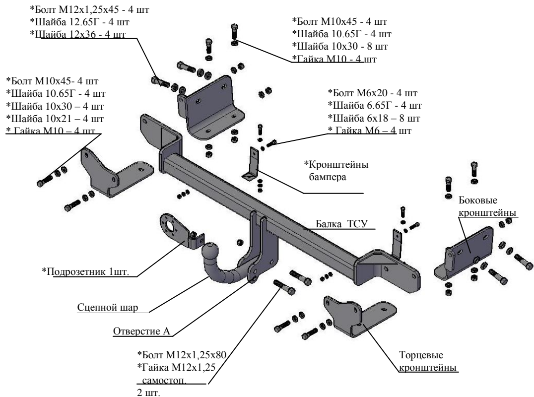
Рис.1 Тягово-сцепное устройство 7240
